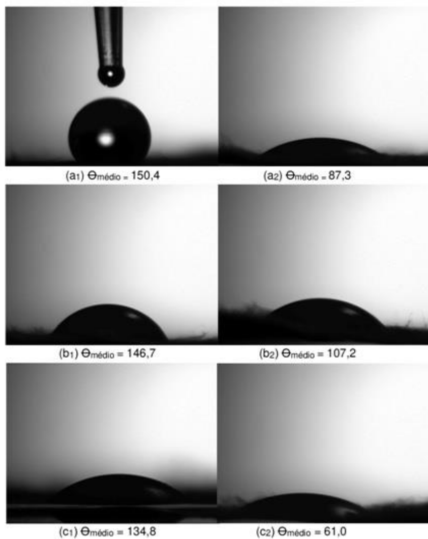
Figura 4: Ângulo de contato das nanofibras de zeína com 30% de óleo essencial de tomilho (a 1 , a 2 ), zeína com 40% de óleo essencial de tomilho (b 1 , b 2 ) e zeína com 60% de óleo essencial de tomilho (c 1 , c 2 ).
