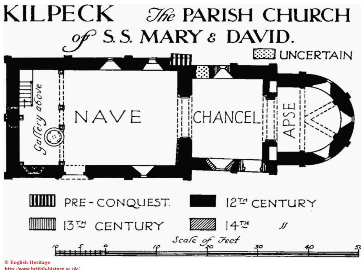
Imagem 13: Planta da Igreja de Kilpeck. Fonte: The Royal Commission on Historical Monuments of England.
